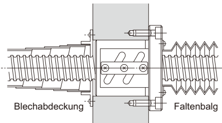
Blechabdeckung für Kugelgewindetrieb
