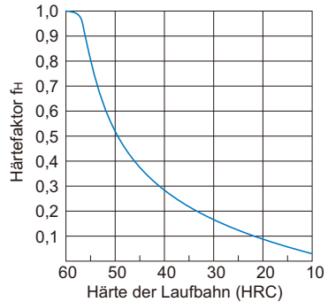
Abb. 1 Härtefaktor ( f_H )
