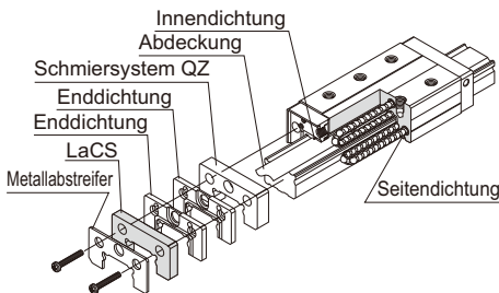
Abdichtungsoptionen für Linearführung
