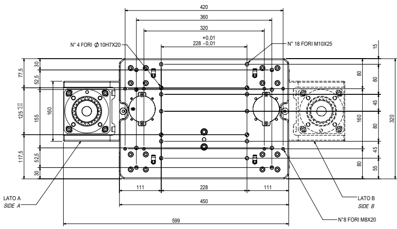
Tipologia interfaccia riduttore ② Gearbox interface type Kit IF85
