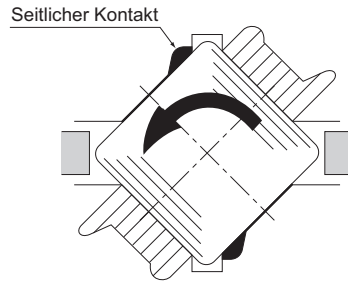
Asymmetrische Lastverteilung mit Blechkäfig (herkömmliches Lager)
