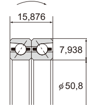
Schrägkugellager
