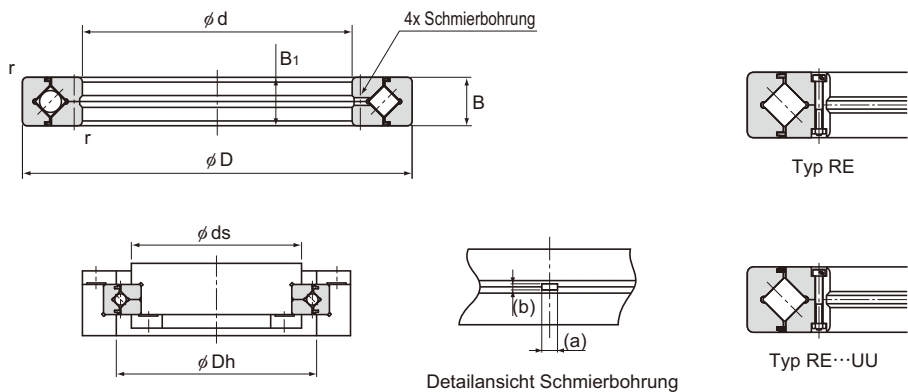
Detailansicht Schmierbohrung
