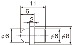
NP6×5
