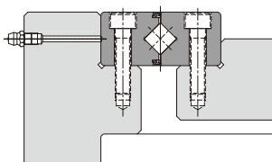
Abb. 3 Montagebeispiel für Typ RU
