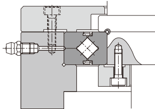
Montagebeispiel RB - 1
