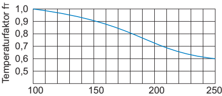
Abb. 1 Temperaturfaktor (f T )
