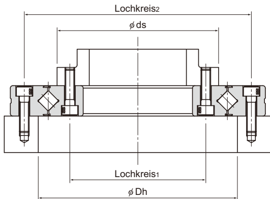
Typ RU...UU
