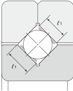
Mit Distanzstücken
