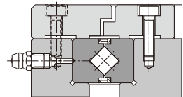
Montagebeispiel RB - 2
