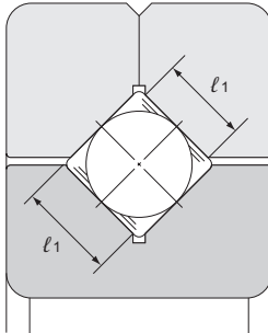
Mit Distanzstücken
