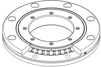
Typ RU
