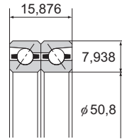
Schrägkugellager
