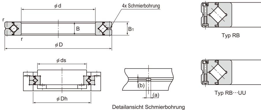
Detailansicht Schmierbohrung
