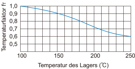
Abb. 1 Temperaturfaktor (f T )
