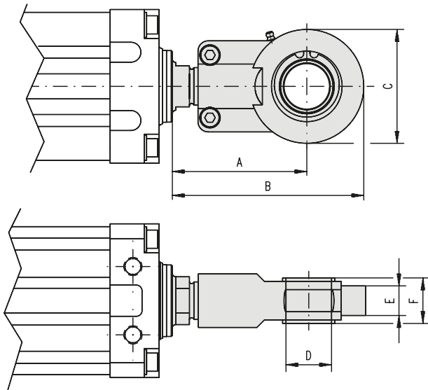
Typ M
