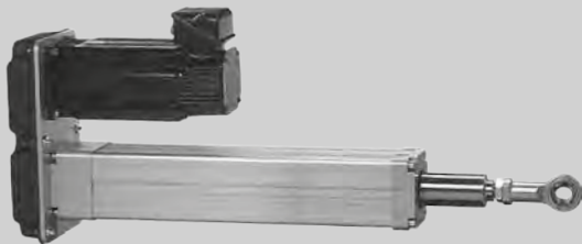
ECT130
