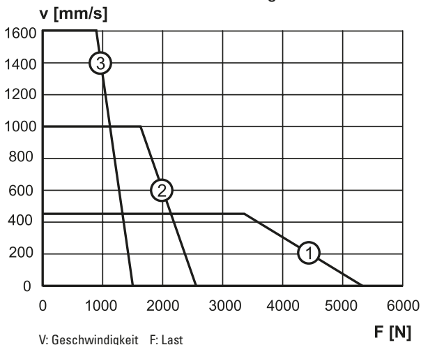
Verhältnis Geschwindigkeit/Last
