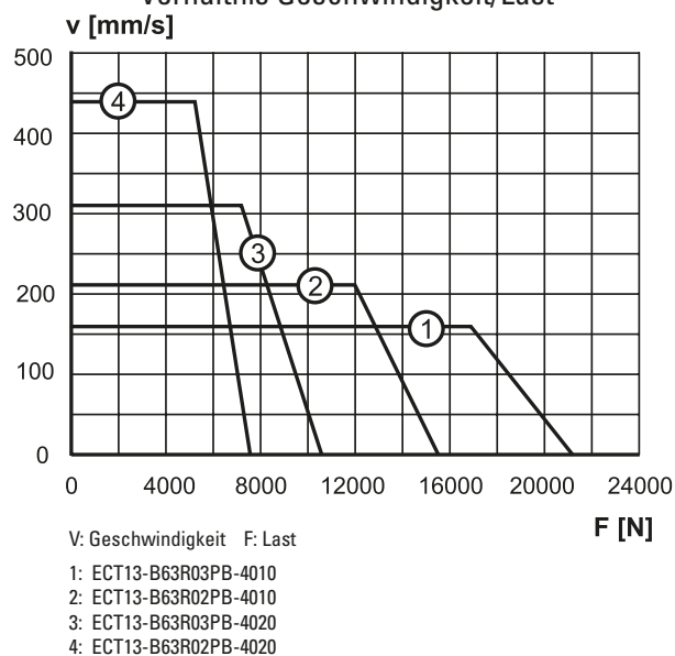
Verhältnis Geschwindigkeit/Last
