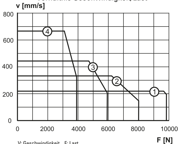
Verhältnis Geschwindigkeit/Last
