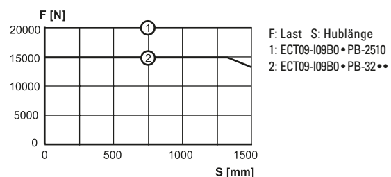
Verhältnis Knicklastgrenze / Hub
