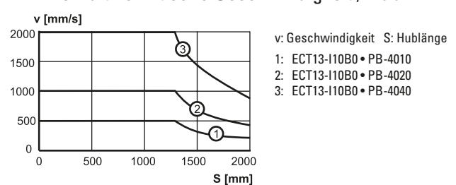
Verhältnis kritische Geschwindigkeit / Hub
