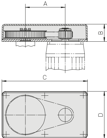
BGM09/41/81 – OHNE OPTIONALEN GABELKOPF
