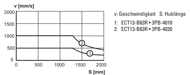
Verhältnis kritische Geschwindigkeit / Hub
