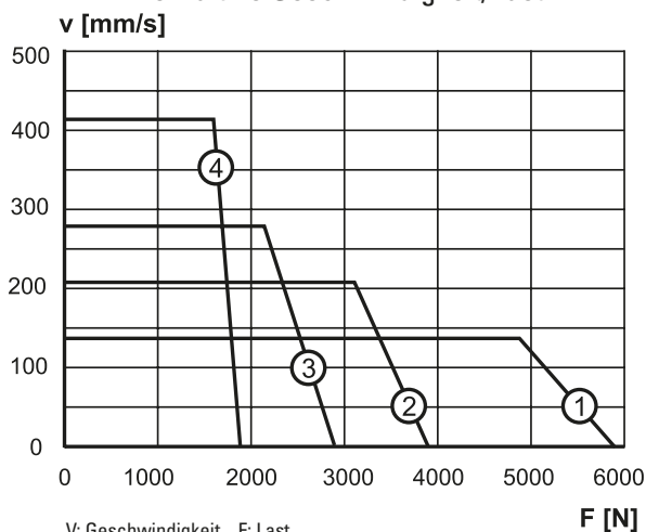
Verhältnis Geschwindigkeit/Last
