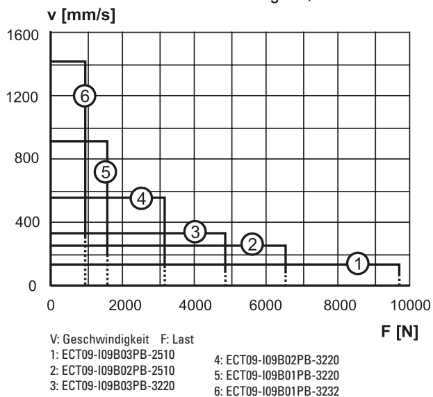
Verhältnis Geschwindigkeit/Last
