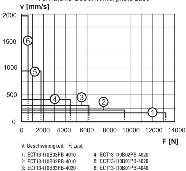
Verhältnis Geschwindigkeit/Last
