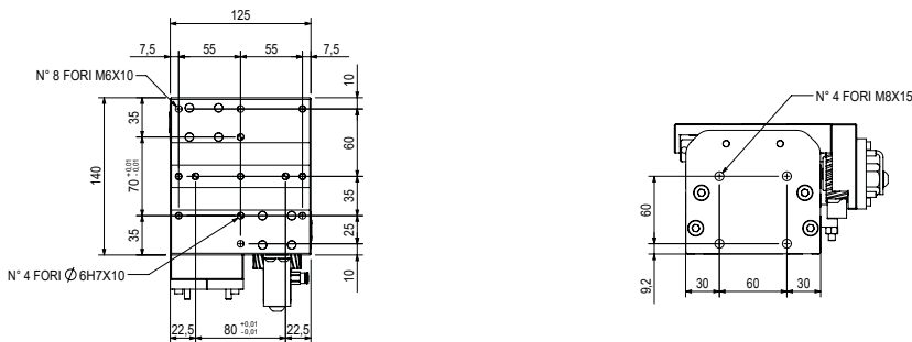
Tipologia interfaccia riduttore (2) Gearbox interface type Kit IF55
