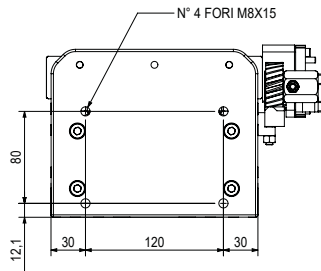
Tipologia interfaccia riduttore ② Gearbox interface type Kit IF75
