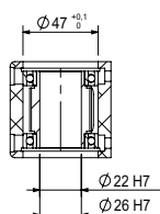
SEZ. C-C
