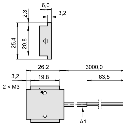
A1: Kabel 2 \times 0,12 \text{ mm}^2
