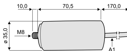
A1: Kabel 2 \times 0,75 \text{ mm}^2
