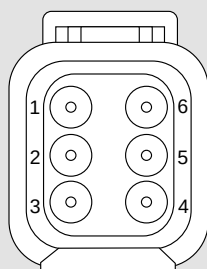
Rückansicht des Deutsch-Steckers
