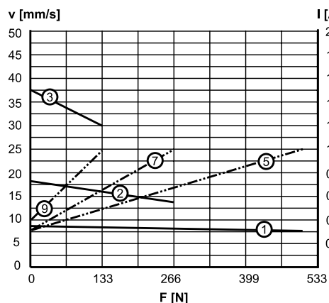
050, Q-Version Geschwindigkeit/Strom vgl. mit Last
